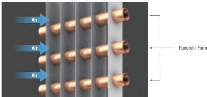
Rundrohr-Wärmetauscher
