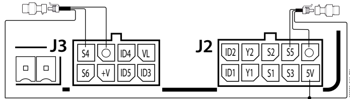
Fühler 4...20 mA/digitale Eingänge
