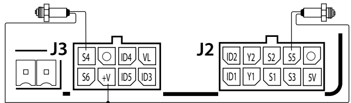
Ratiometrische Druckfühler 0...5V
